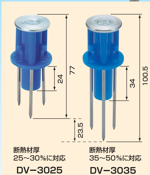
DV-3025 (断熱材料25-30mm用)
