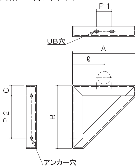
形状②：三角ブラケット
