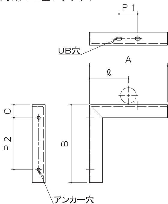
形状①：L型ブラケット
