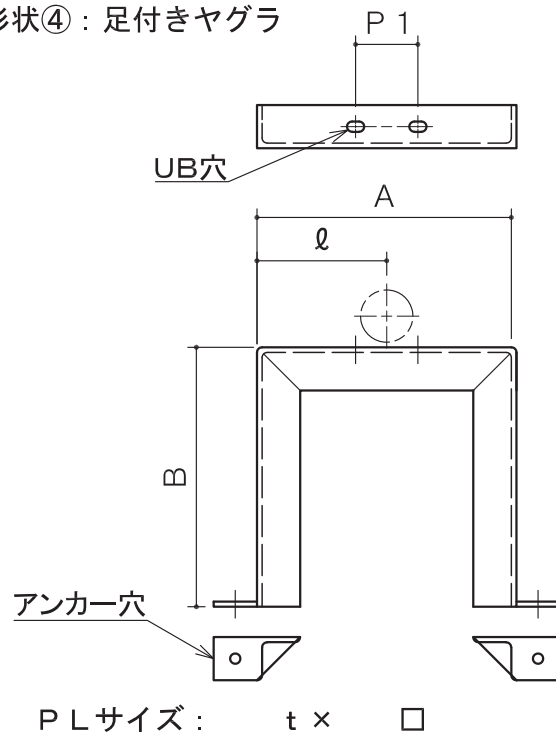
各架台 寸法表
